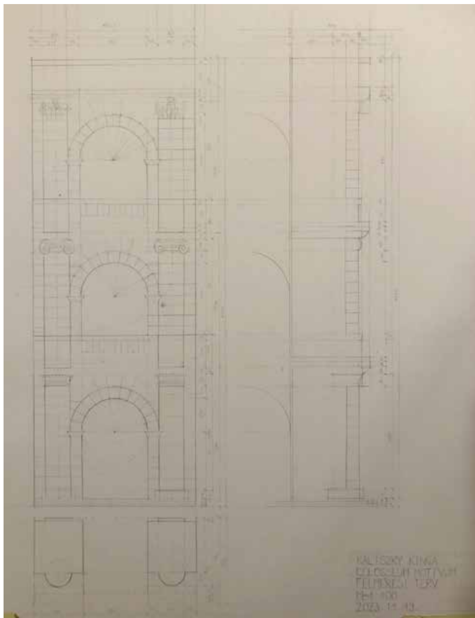
A Colosseum-motívum felmérési terve:
