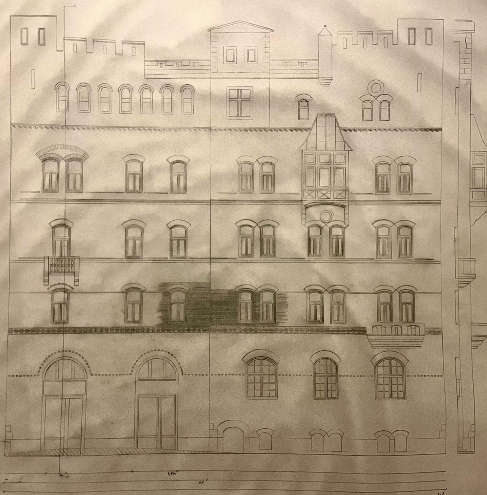
Felmérési rajz
