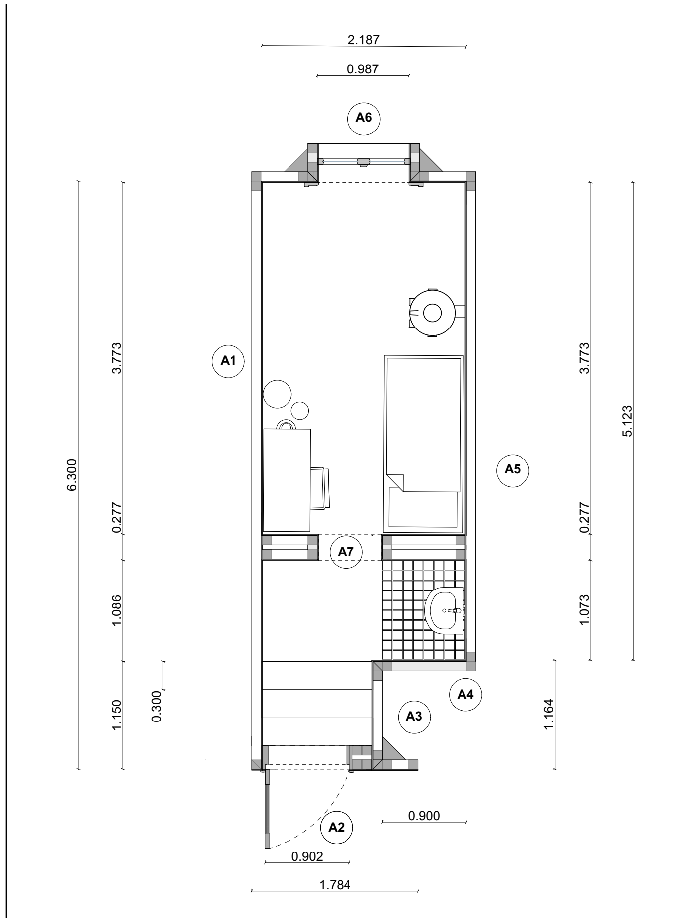
Ötödik pecsét, Keszei-zug Tyler Szonja Alaprajz M: 1:25
